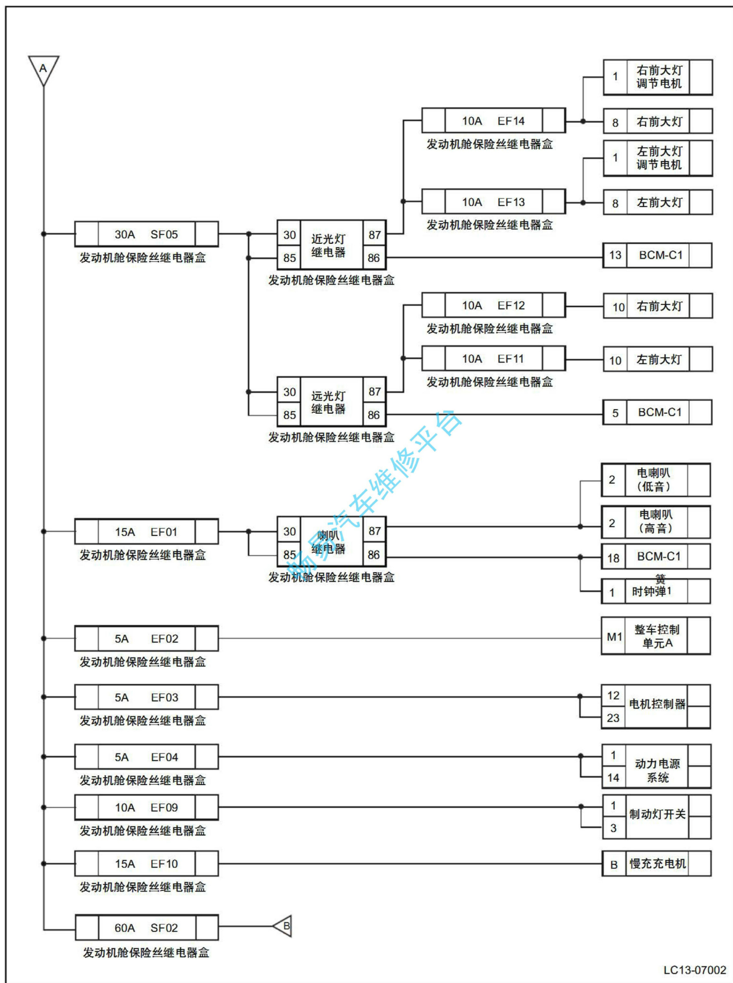
电源配置电路图 2
