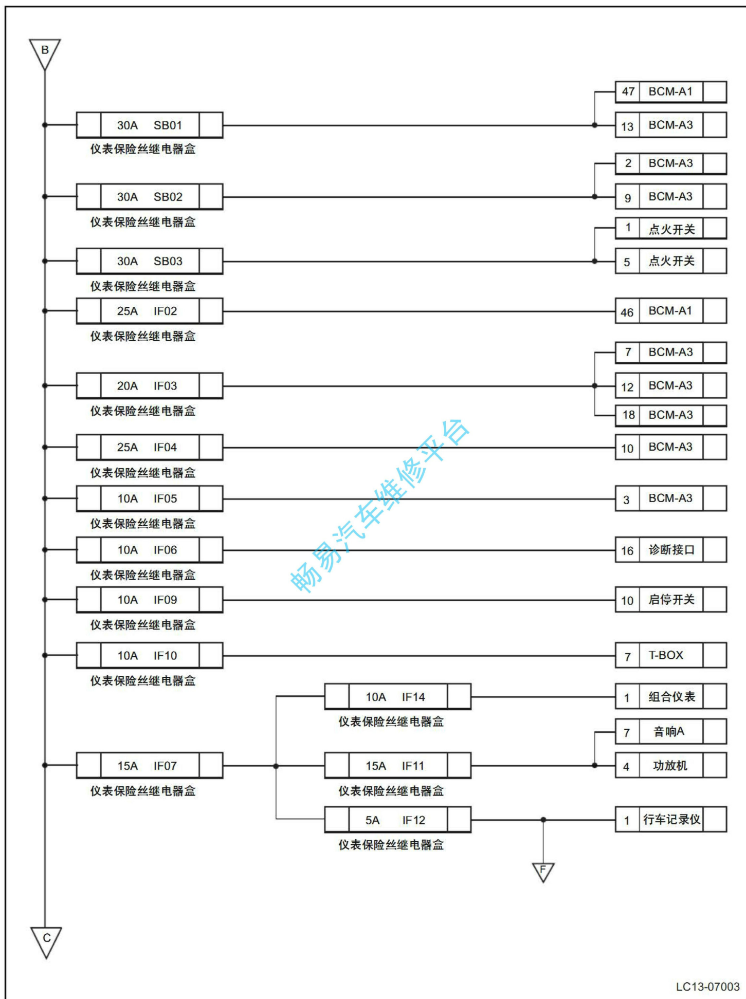
电源配置电路图 3
