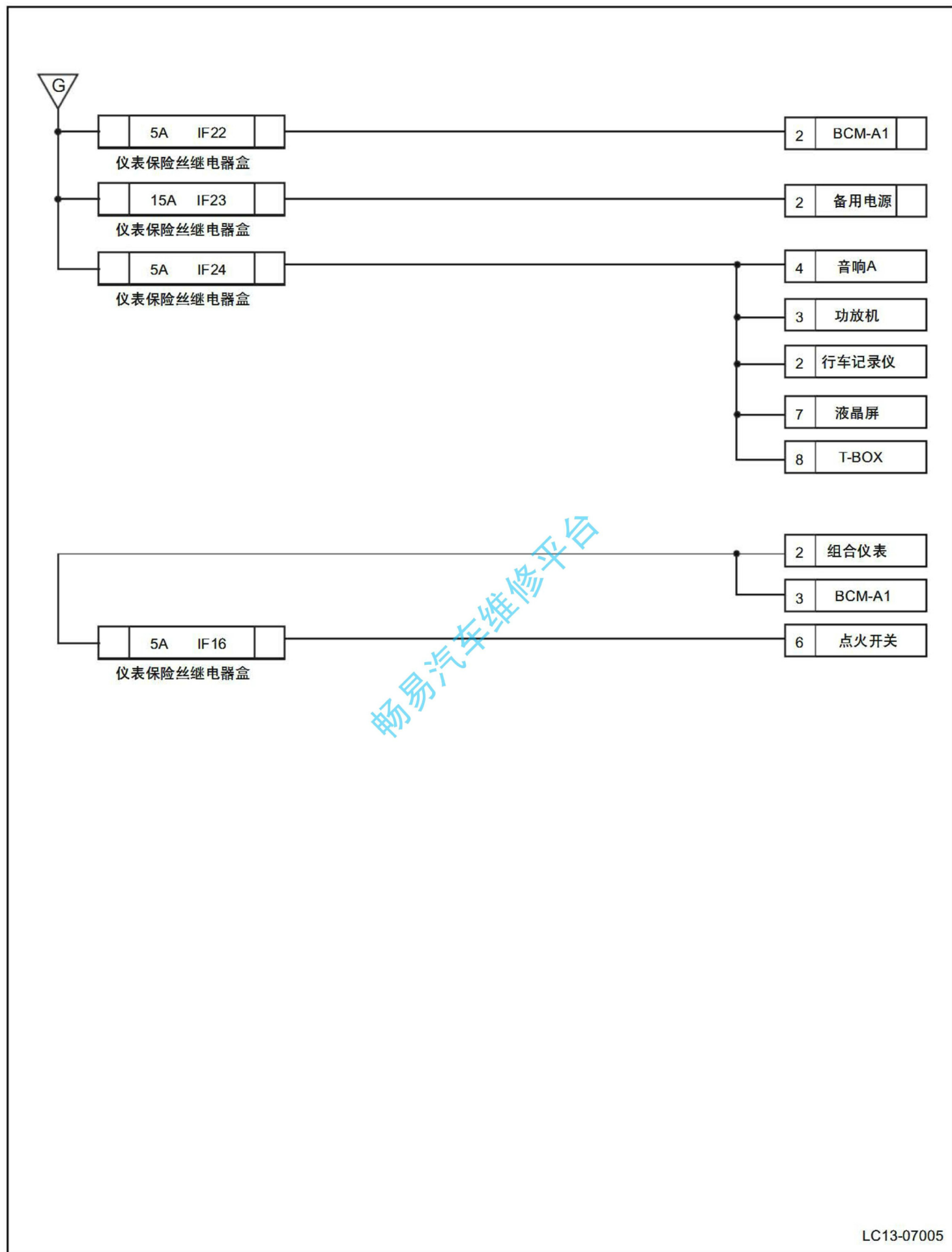
电源配置电路图 5
