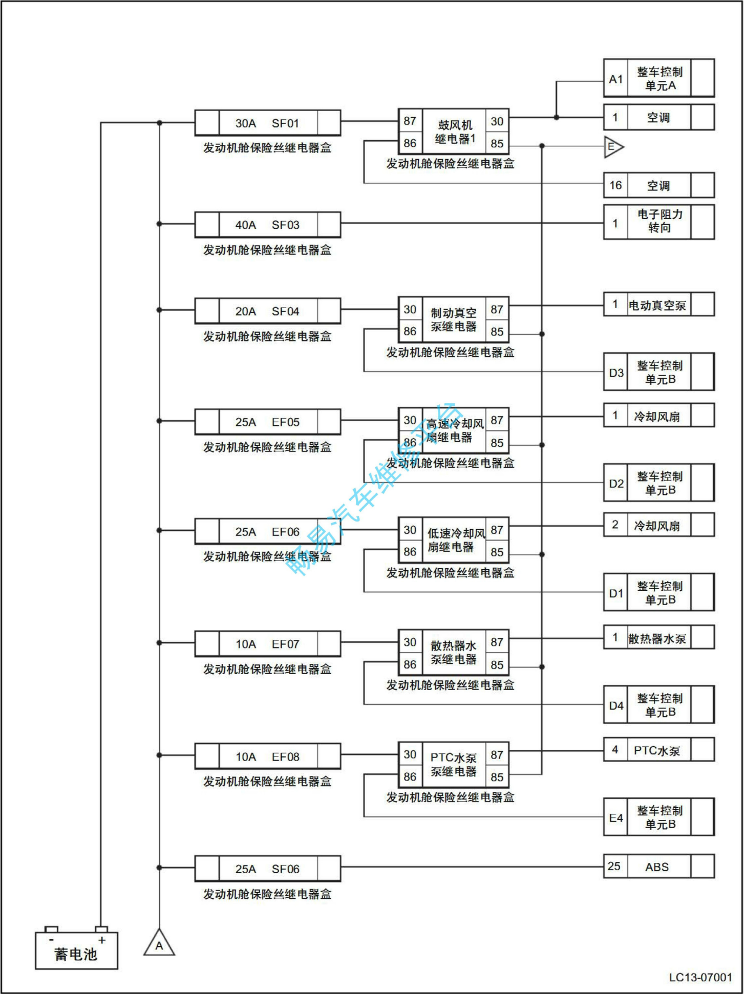
电源配置电路图 1
