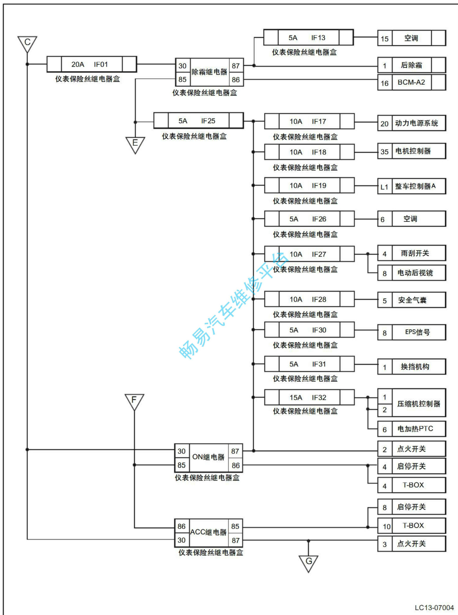
电源配置电路图 4
